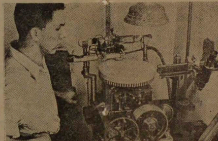
3) Máquina de grabación, complicado mecanismo de alta precisión accionada por la fuerza de gravedad para obtener la más rigurosa exactitud en la veloci- dad. La "Cera" está lista para recibir la incisión de la aguja grabadora la cual es de zafiro.
