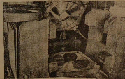
6) Prensa de fabricación donde se acondicionan las matrices y sus respectivas etiquetas. Un bloque de "pasta" se apli- ca a la prensa, se cierra ésta bajo una presión hidráulica de varias toneladas y al abrir... ¡Nace un nuevo Disco Victor!
